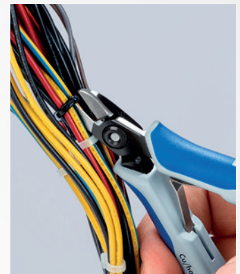
Alle Kanten am Zangenkopf sind speziell verrundet – unbeabsichtigte Beschädigungen der Isolierung werden so vermieden
