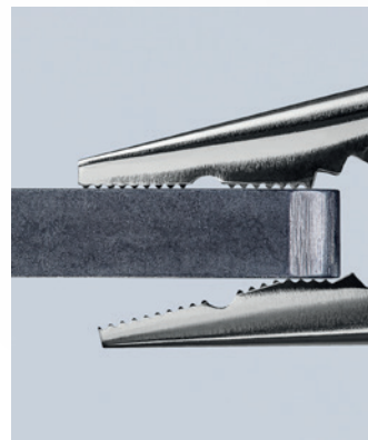
Spitz-Kombizange: ideal zum Greifen flacher Teile dank einseitig konvexer Greiffläche
